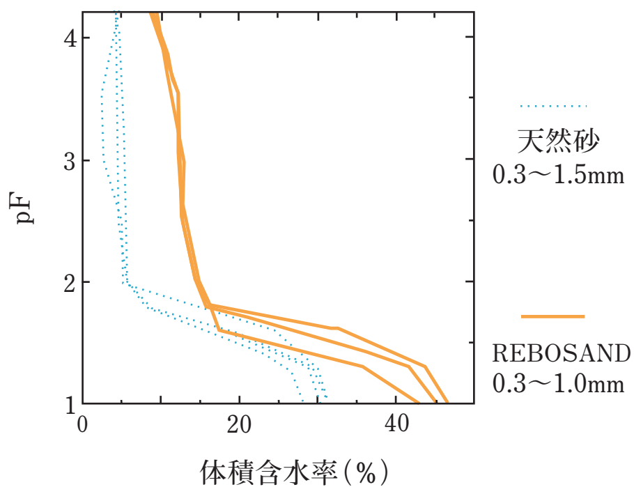
図2 pF 試験(保水性試験)の測定結果(試料数：天然砂のみ4,その他は3)
